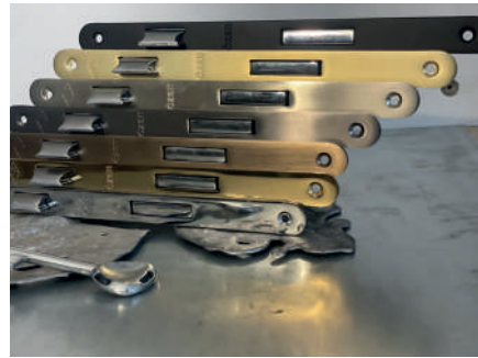
Backset
